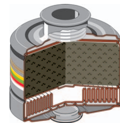
Dräger X-plore® Rd40 Filter: cross-section
